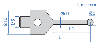
M5 styli (mm)
